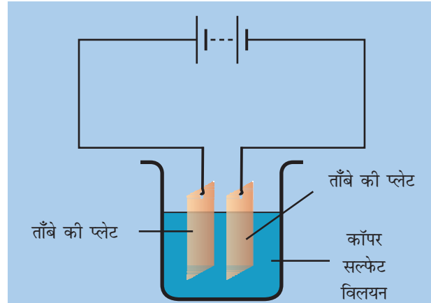
चित्र 11.7 : विद्युतलेपन दर्शाता सरल परिपथ।
